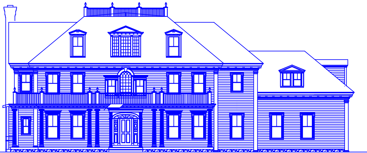
ELEV. "B"
